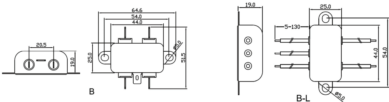
外形尺寸 Outline Dimensions(mm)
